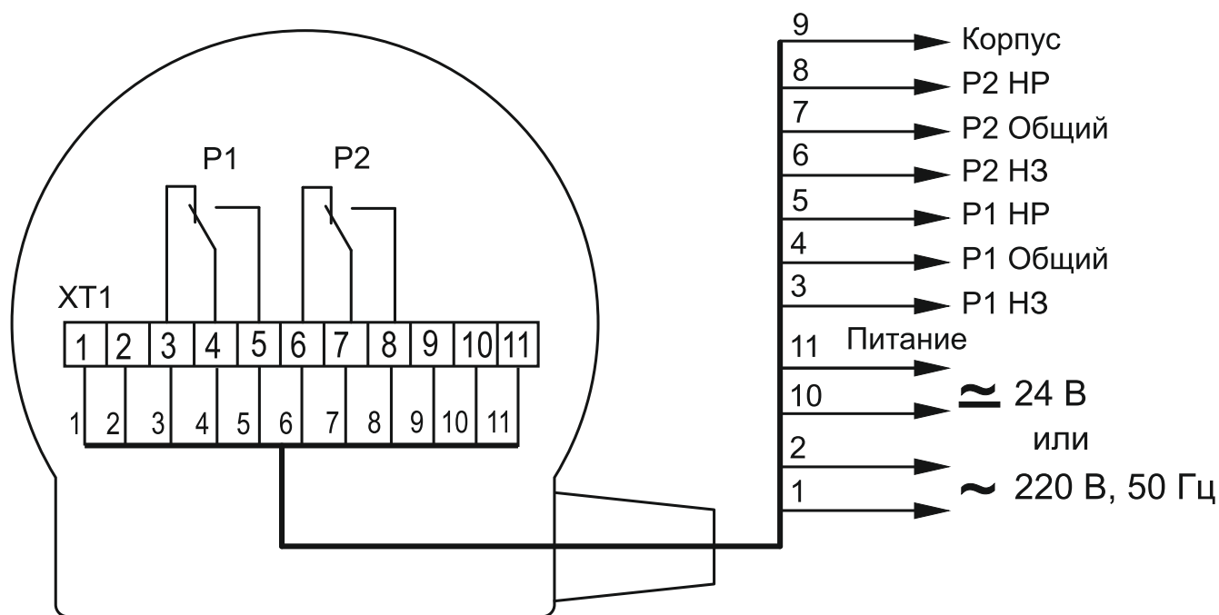
Рисунок 3 – Схема электрическая подключения
